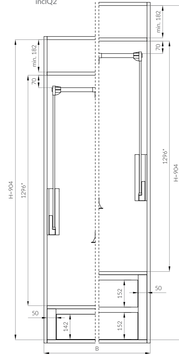
Габариты шкафа Wardrobe (cabinet) dimensions
