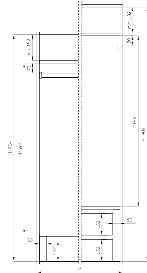
Габариты шкафа Wardrobe (cabinet) dimensions
