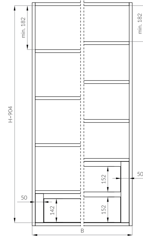
Габариты шкафа Wardrobe (cabinet) dimensions
